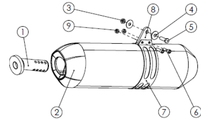
Opción Abrazadera
